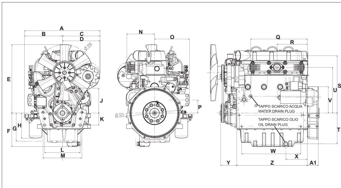
DIMENSIONI mm - MESURES mm - DIMENSION mm - EINBAUMAßE mm - DIMENSIONE mm - DIMENÇÕES (mm)
