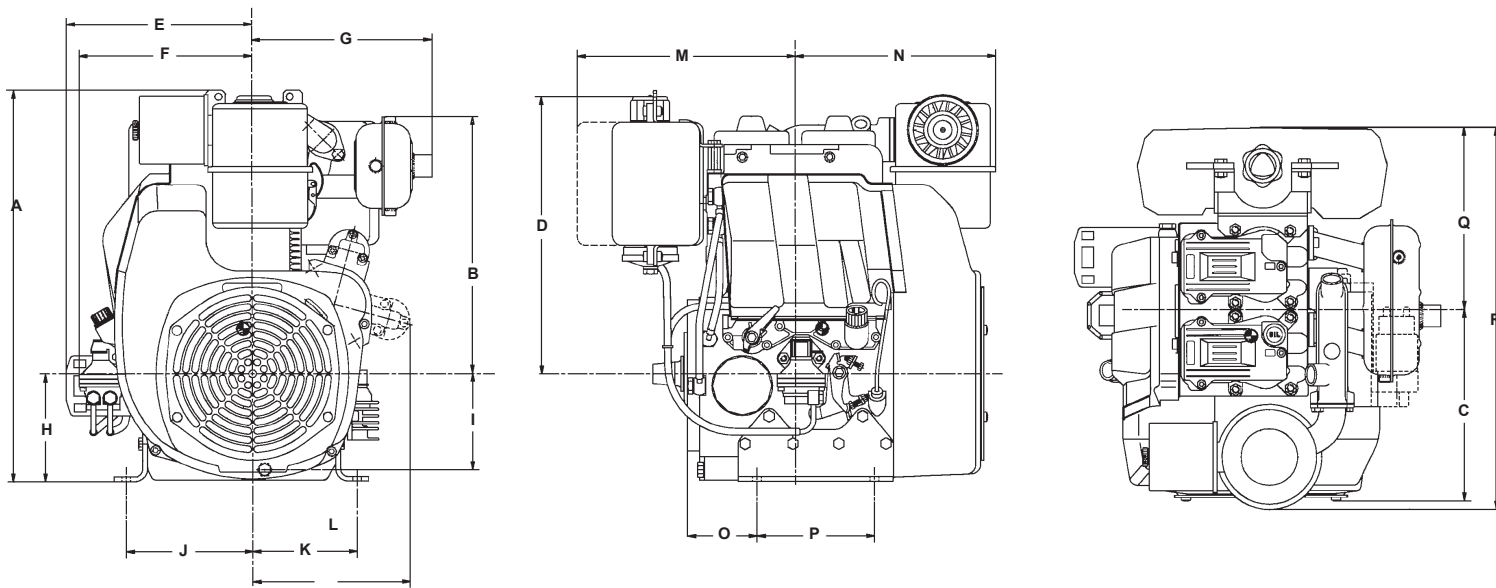
DIMENSIONI (mm) - MESURES (mm) - DIMENSION (mm) - EINBAUMÄßE (mm) - DIMENSÃO (mm) - DIMENÇÕES (mm)
